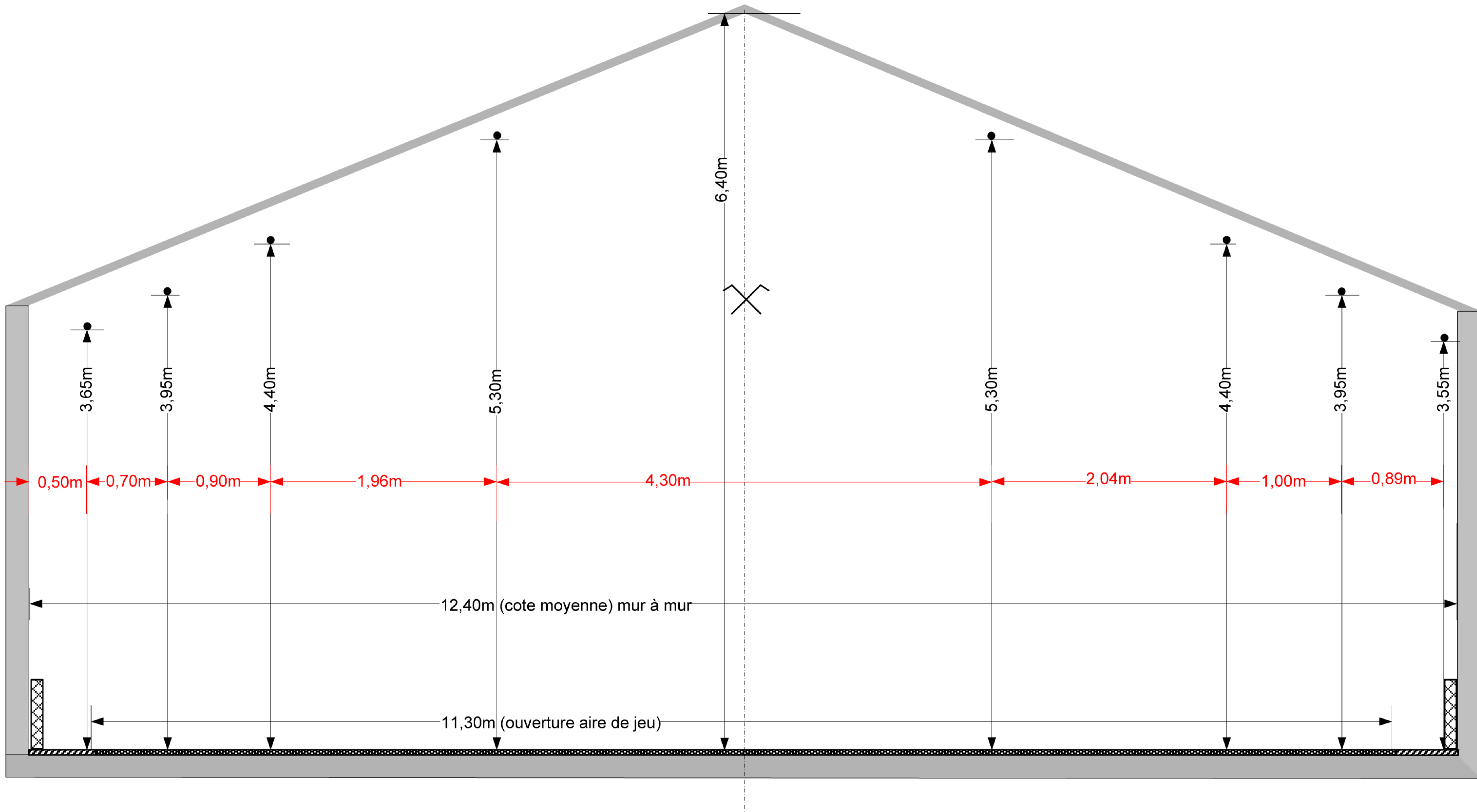
Le Colombier Plan coupe hauteurs porteuses latérales ECH : 1/50ème 20 rue Marie-Anne Colombier - 93170 Bagnolet Téléphone : 01.43.60.72.81
